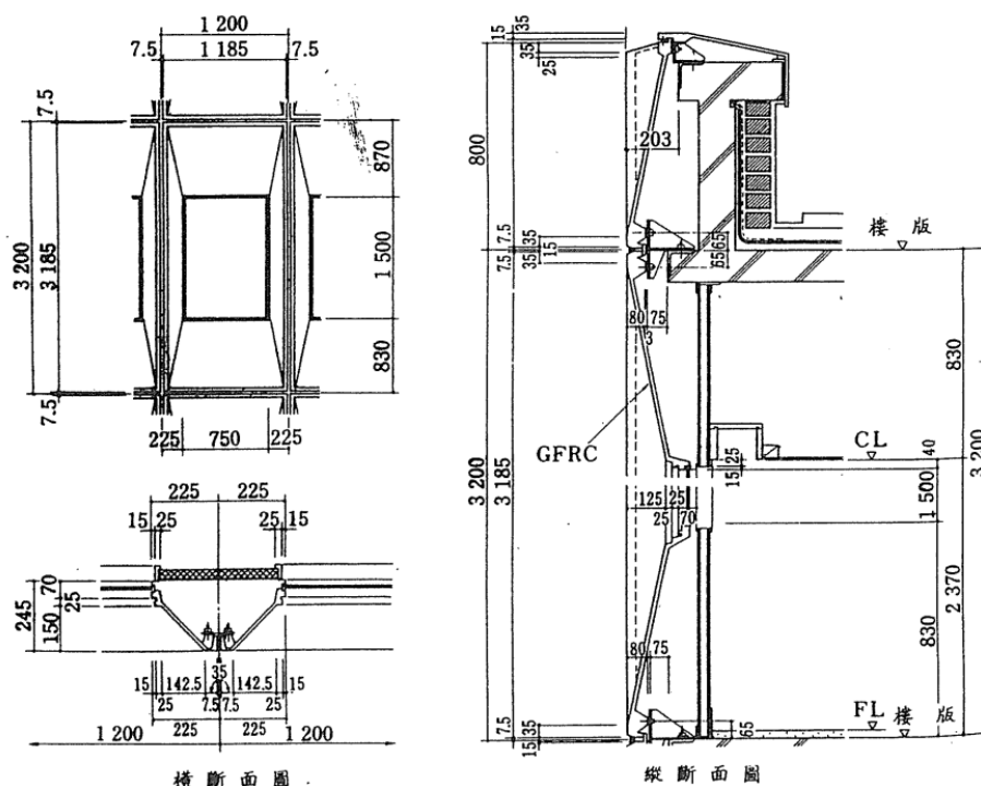
圖 R7.37 GFRC 帷幕牆圖例(單位：mm) [7.5]
