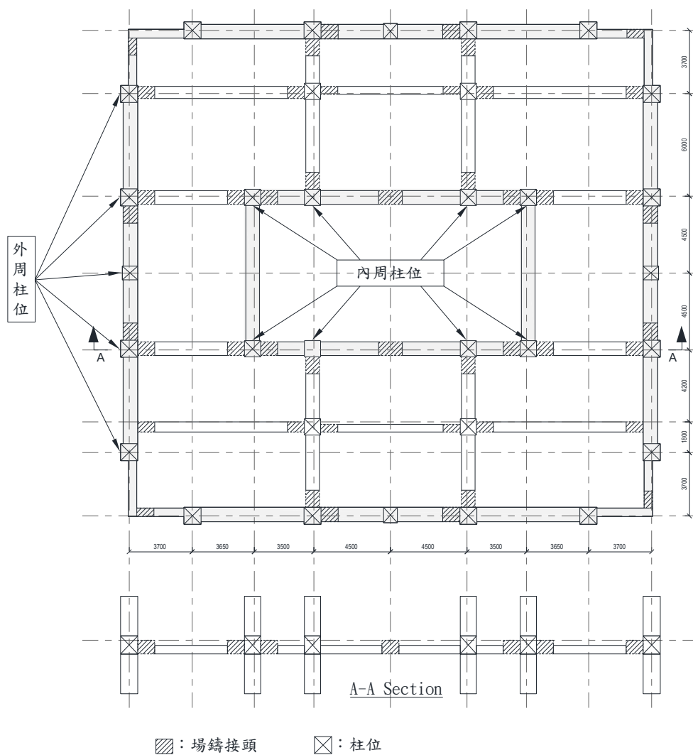
圖 R7.7 預鑄特殊抗彎矩構架工法例(單位：mm)
