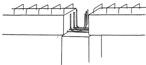
(1) L 形搭接
