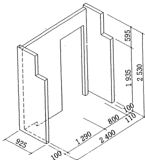
圖 R7.34 預鑄立體牆圖例(單位：mm) [7.5]
