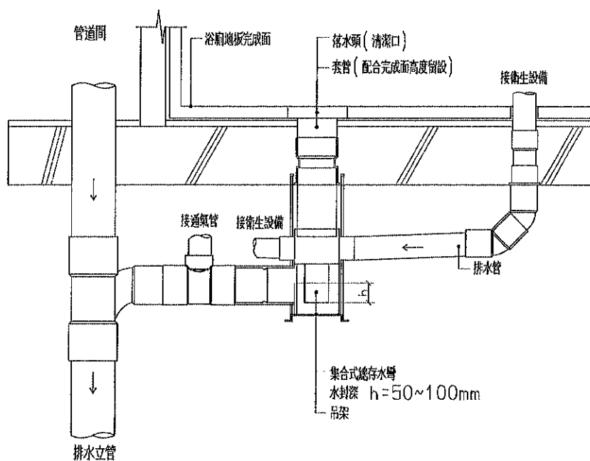
圖4-18-4 隔層懸吊式剖面示意圖
