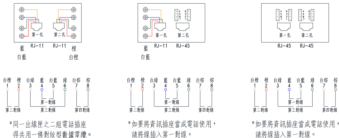
插座配線圖
