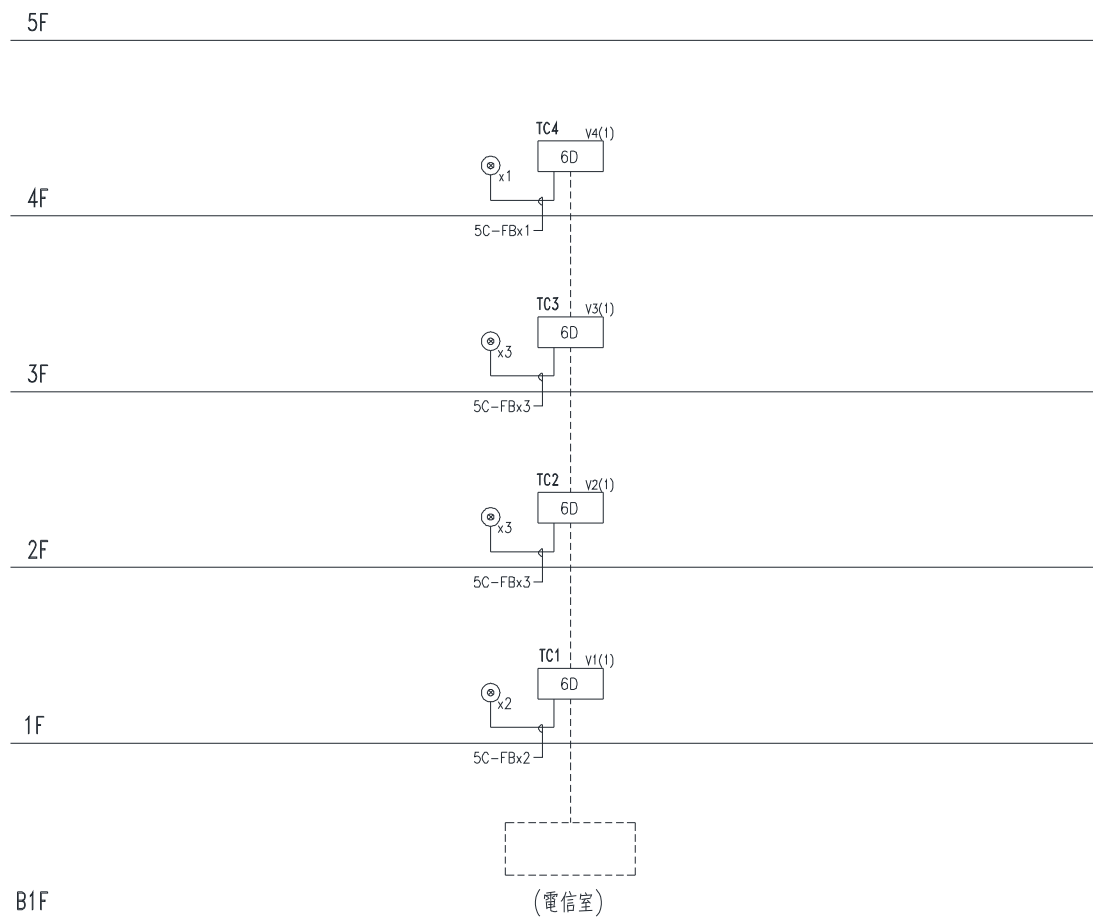
圖17-24 設計範例(六)電視電纜昇位圖
