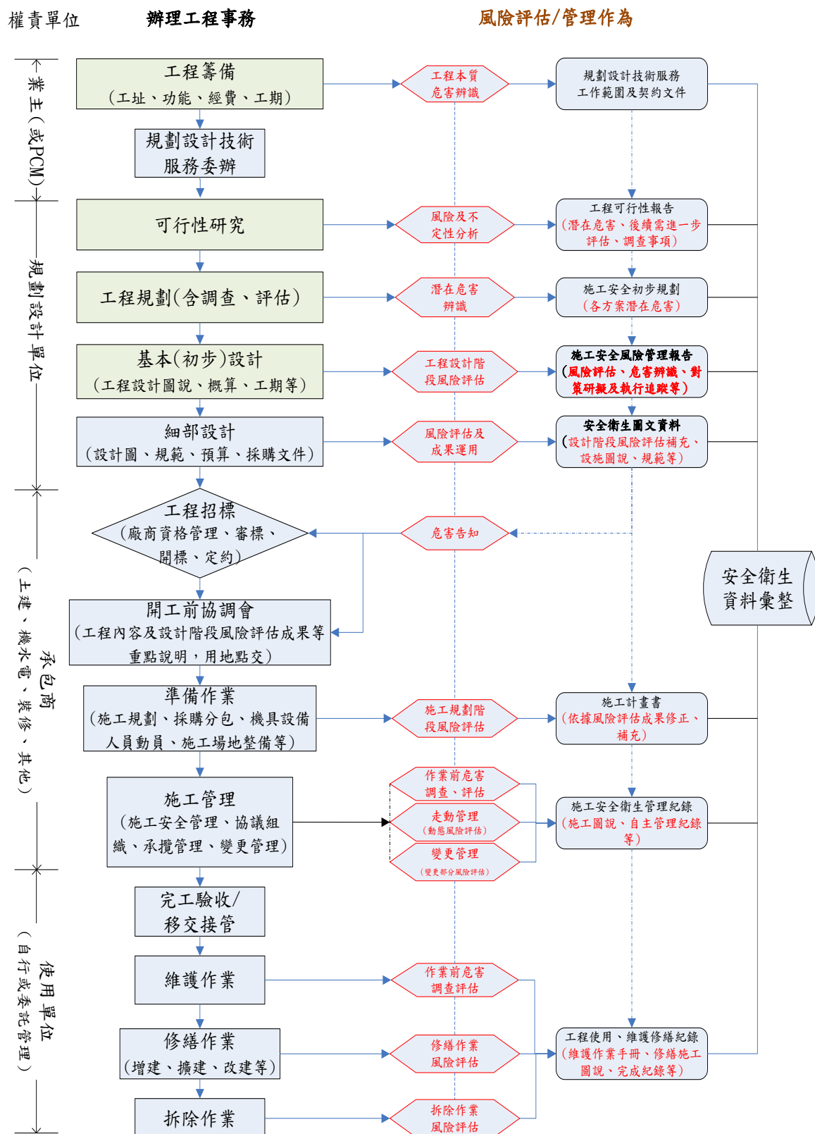
圖 24. 營造工程全生命週期施工風險管理資訊傳遞流程
