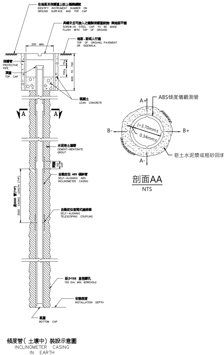
圖 A-2 土層內傾度管安裝示意圖
