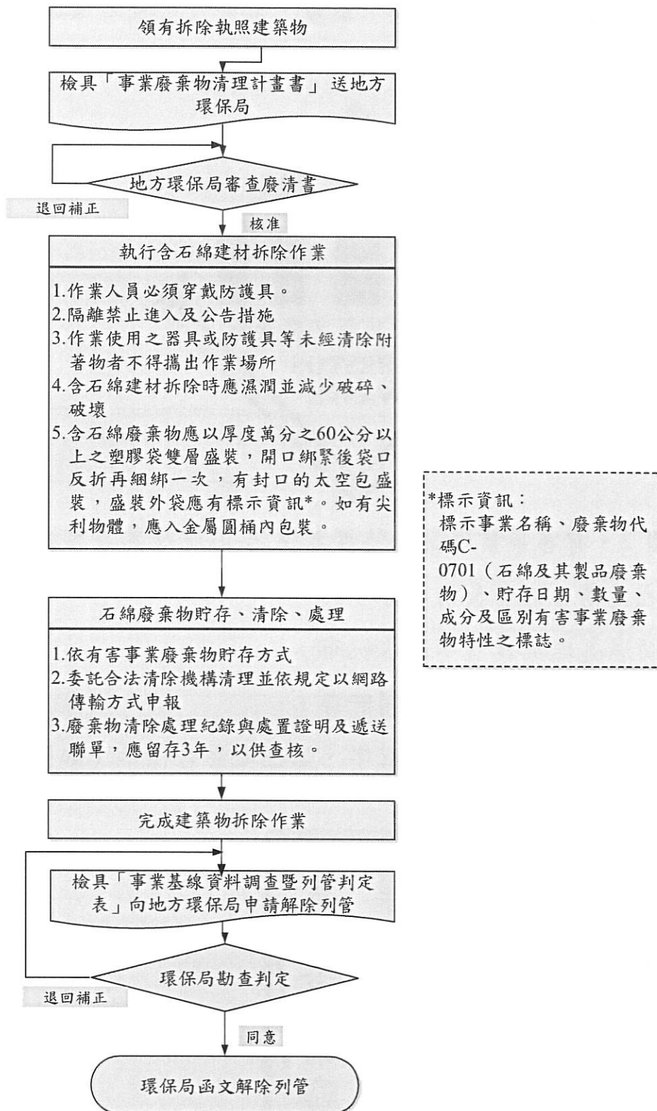
圖 1、含石綿之建材拆除後之廢棄物處理作業流程
