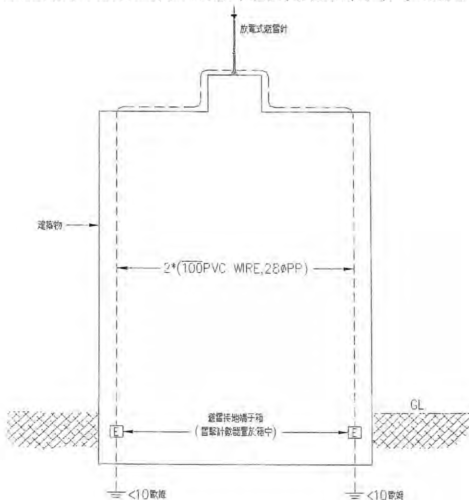
放電式避雷針裝置架構圖（一）
