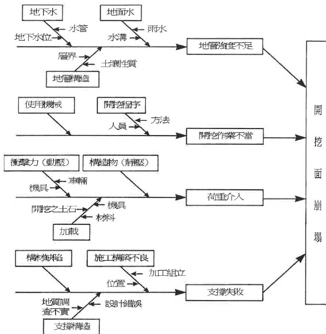
圖3.2 開挖面崩塌之災害要因圖
