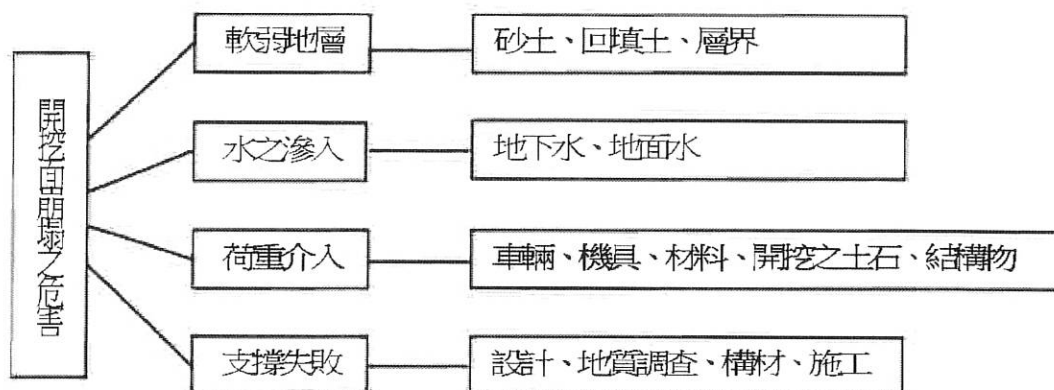
圖3.1 開挖面崩塌之危害狀況引導圖
