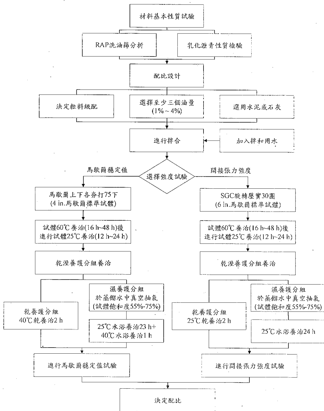
圖 A.1 冷拌再生乳化瀝青混凝土配合設計流程圖
