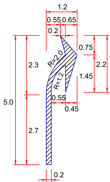
27 弧形箭頭(1) §188 (數量:3m 2 )
