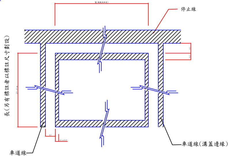
34 機慢車停等區線§174-2 (寬x2x0.2+長x2x0.1~0.15)
