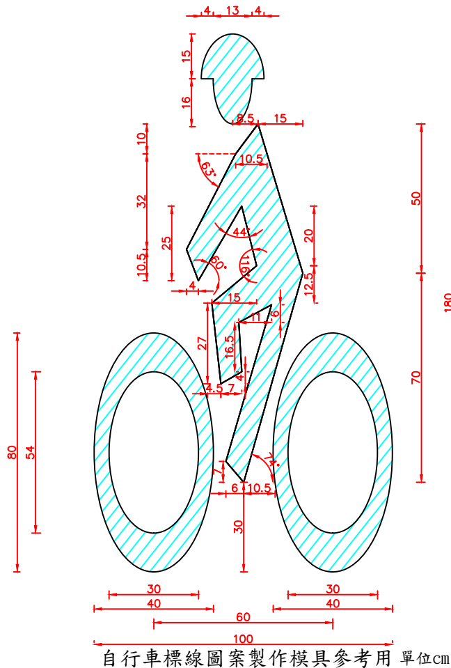
36 路面熱拌自行車標線 數量：(1.8x1)x1.5=2.7m 2
