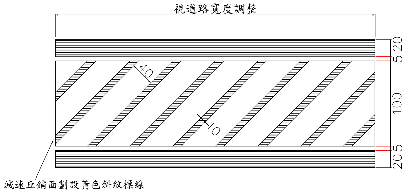
減速丘正視圖
