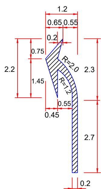
28 弧形箭頭(2) §188 (數量:3m 2 )
