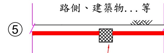
禁止(臨時)停車標線劃設示意圖 註:未在本示意圖範圍內,請比照辦理
