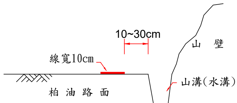
禁止(臨時)停車標線劃設示意圖 註:未在本示意圖範圍內,請比照辦理
