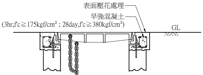
完成示意圖(四)
