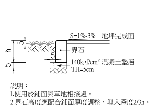
鋪面收邊詳圖(一) NTS Unit:cm
