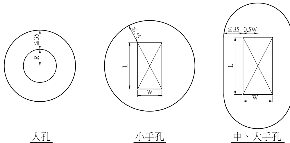
圓形切割方式示意圖
