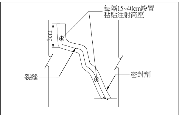
平面示意圖
