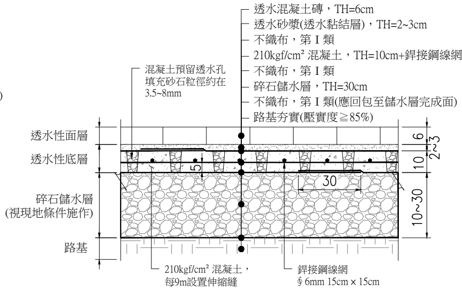
透水磚鋪面(混凝土底層)詳圖 NTS Unit:cm
