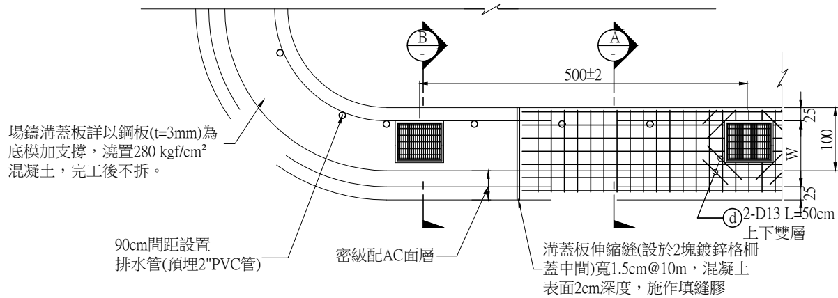
箱涵式側溝(場鑄溝蓋版)平面圖 A1 (1:40) A3 (1:80) Unit:cm
