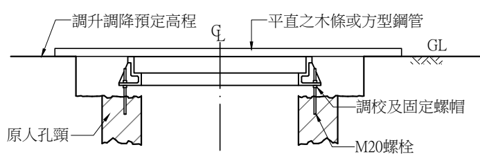
施工中示意圖(二)
