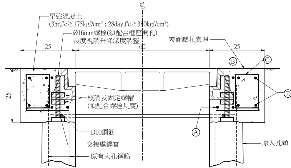
路面人孔調升降剖面圖 3 NTS Unit:cm
