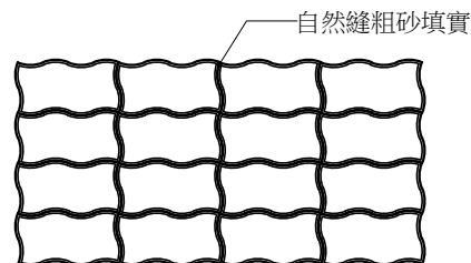
高壓混凝土磚鋪面平面圖(軟底層) A1 (1:10) A3 (1:20) Unit:cm
