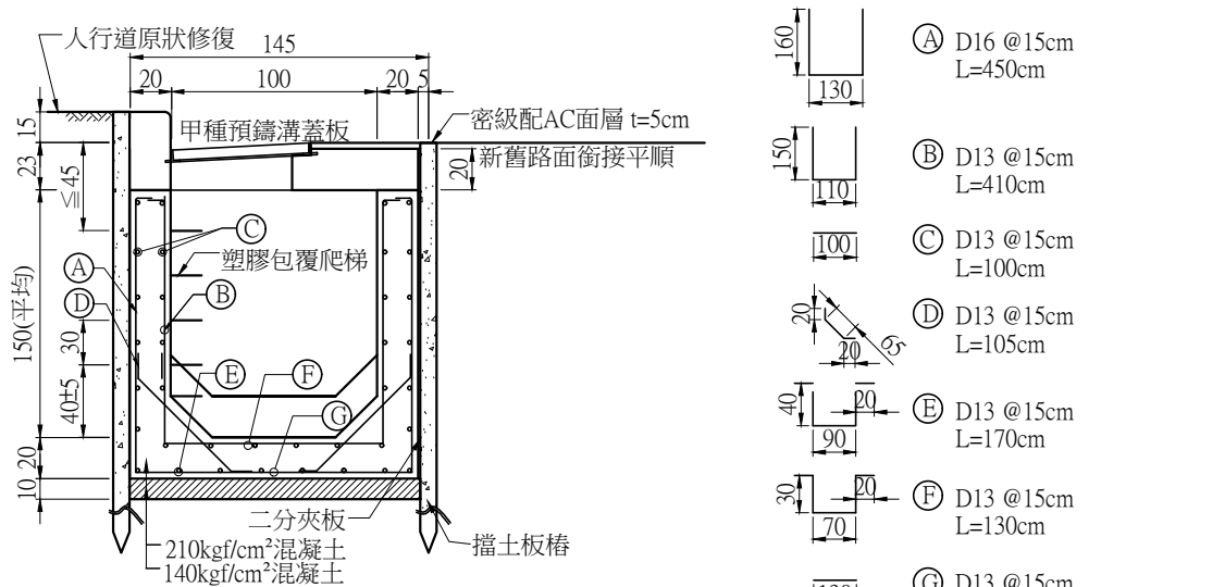
集水井剖面圖 A1 (1:20) A3 (1:40) Unit:cm
