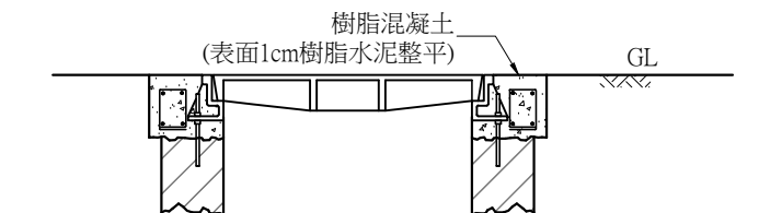
施工中示意圖(四)
