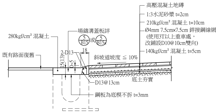
側溝蓋板上方設置 0~5公分緣石之收邊斜坡詳圖 A1 (1:20) A3 (1:40) Unit:cm
