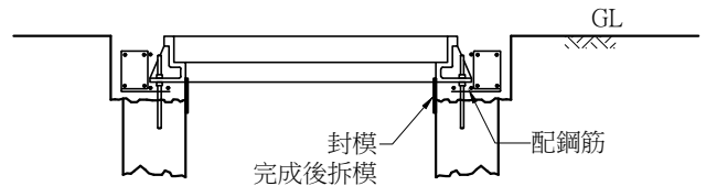
施工中示意圖(三)
