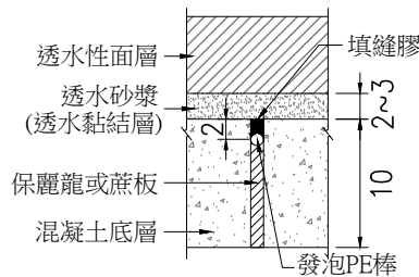
混凝土底層伸縮縫詳圖 NTS Unit:cm
