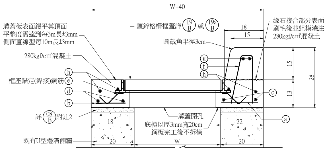
L 2型場鑄溝蓋板剖面圖(板厚13cm) A1 (1:5) A3 (1:10) Unit:cm
