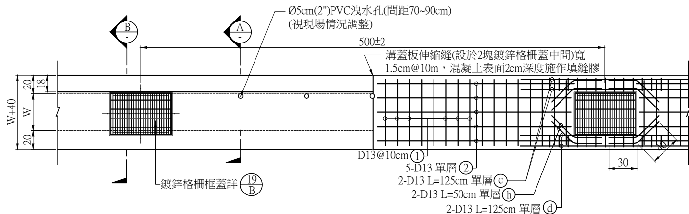
L型溝蓋板平面及鋼筋配置詳圖(板厚13cm) A1 (1:20) A3 (1:40) Unit:cm
