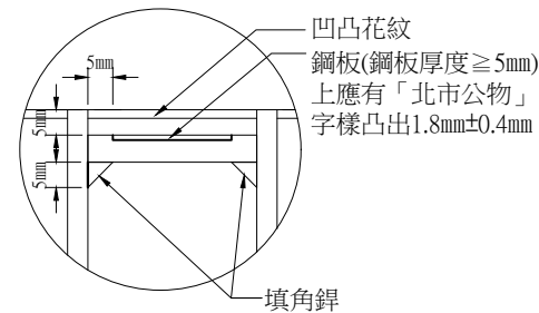
詳圖 A1 (1:1) A3 (1:2) Unit:cm
