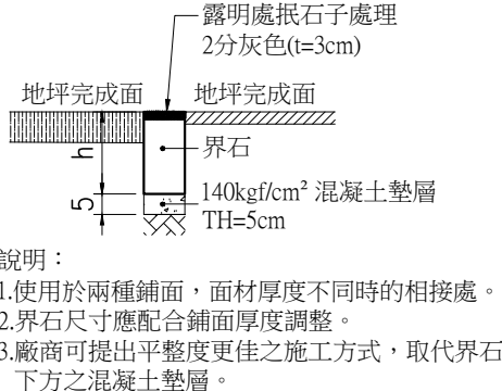
鋪面收邊詳圖(三) NTS Unit:cm ④
