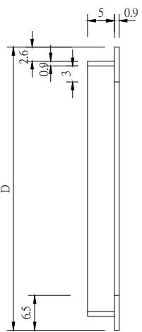
剖面圖 A1 (1:6) A3 (1:12) Unit:cm
