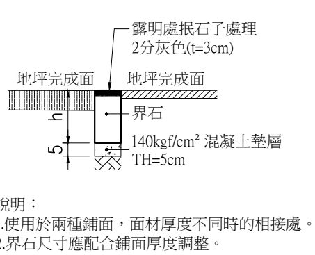
鋪面收邊詳圖(三) NTS Unit:cm
