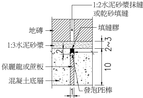
硬底層伸縮縫詳圖 NTS Unit:cm ①
