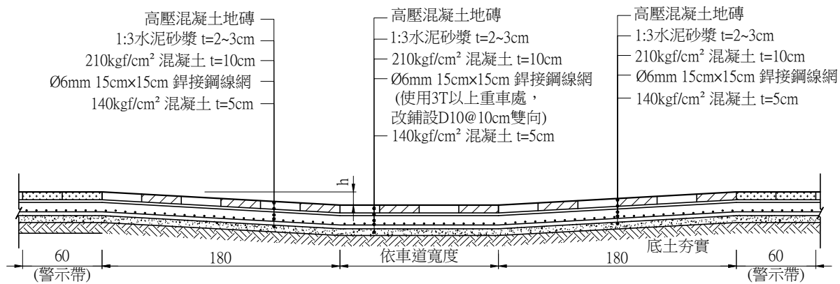
剖面圖 A1 (1:20) A3 (1:40) Unit:cm
