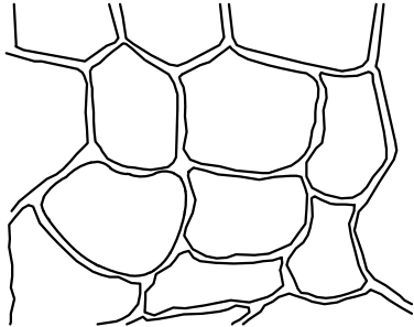
石板鋪面平面圖 A1 (1:10) A3 (1:20) Unit:cm
