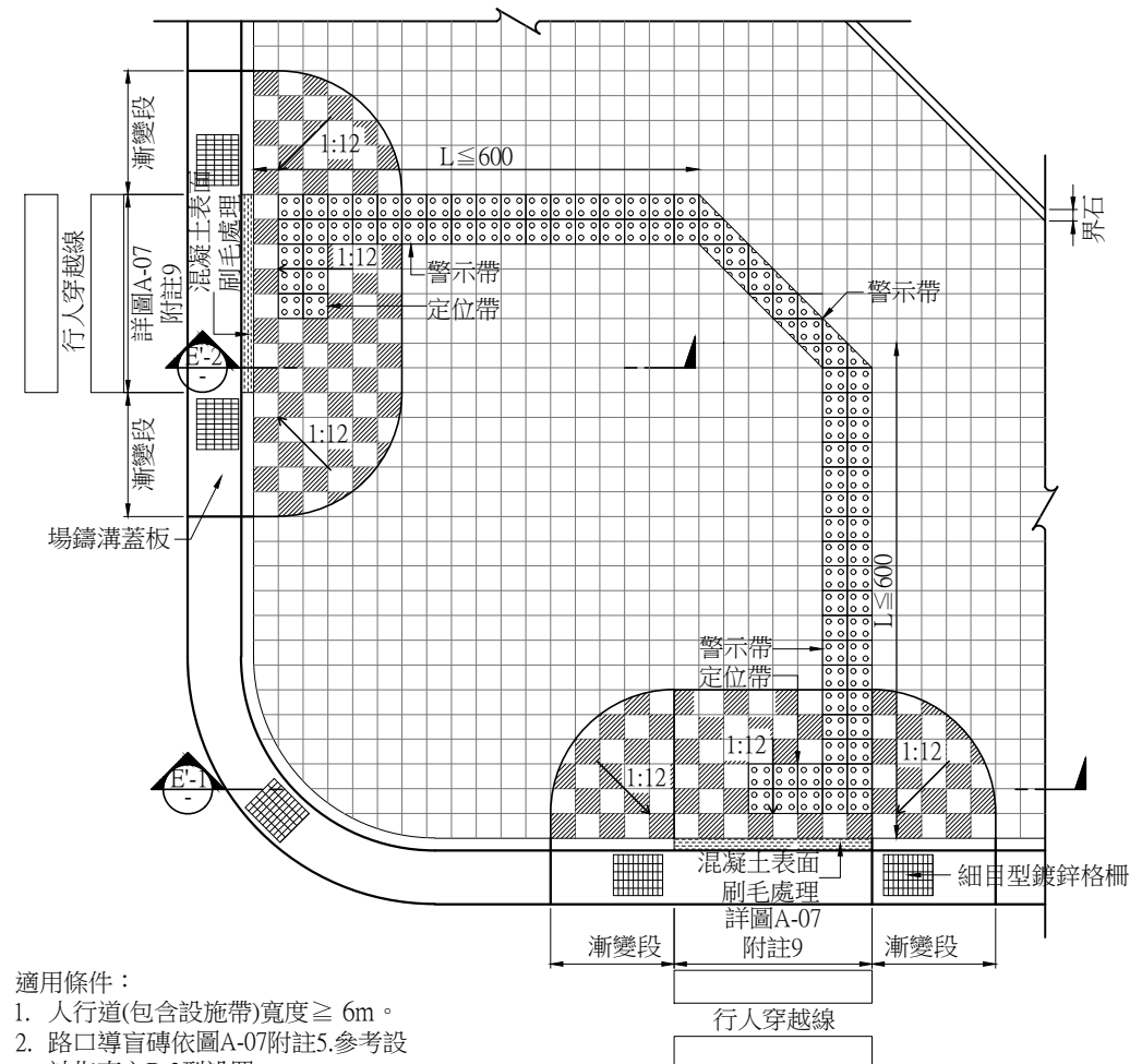
E'型路緣斜坡平面圖
