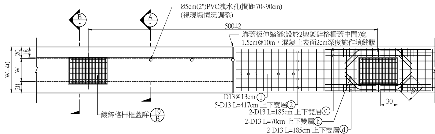
L型溝蓋板平面及鋼筋配置詳圖(板厚15cm) A1 (1:20) A3 (1:40) Unit:cm
