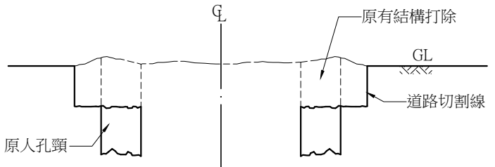
施工中示意圖(一)
