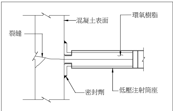
剖面示意圖
