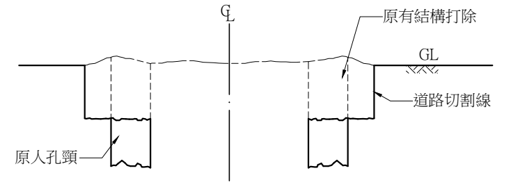
施工中示意圖(一) 6 NTS
