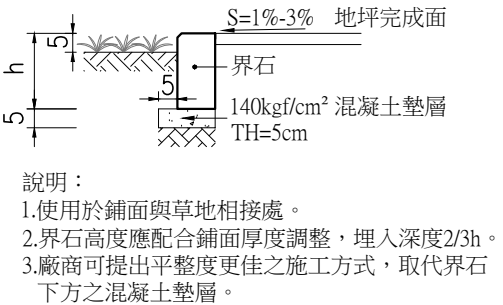
鋪面收邊詳圖(一) NTS Unit:cm ②
