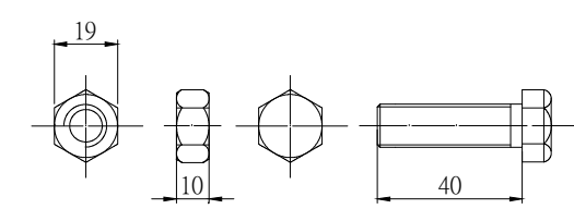
螺絲螺帽詳圖 NTS Unit:mm
