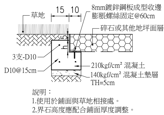
鋪面收邊詳圖(二) NTS Unit:cm
