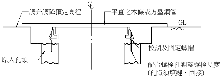
施工中示意圖(二)
