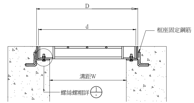
剖面圖 NTS Unit:mm
