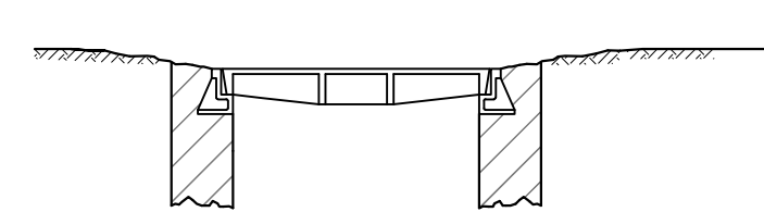
施工前示意圖-凹狀情形(提升)
