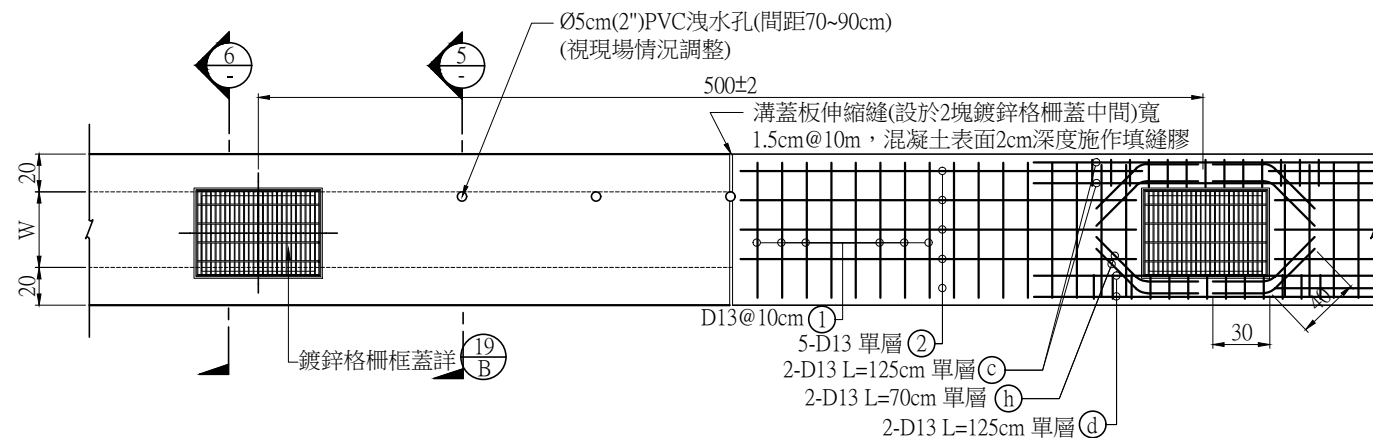
S型溝蓋板平面及鋼筋配置詳圖(板厚13cm) A1 (1:20) A3 (1:40) Unit:cm
