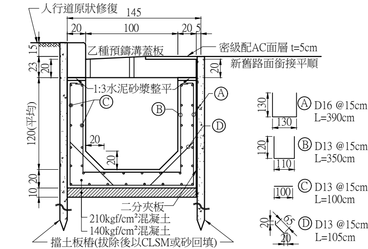
箱涵式側溝剖面圖 A1 (1:20) A3 (1:40) Unit:cm
