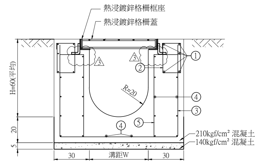
截流溝剖面圖 A1 (1:10) A3 (1:20) Unit:cm
