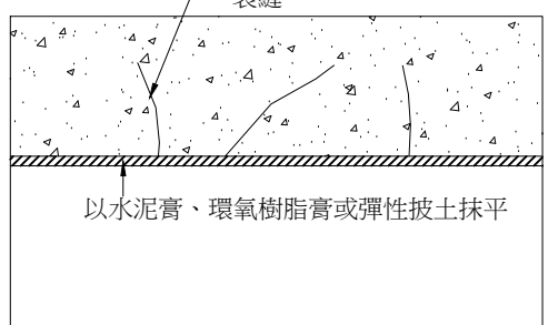
步驟(三)：以水泥膏、環氧樹脂膏或彈性披土填充抹平裂縫
