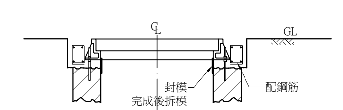
施工中示意圖(三)
