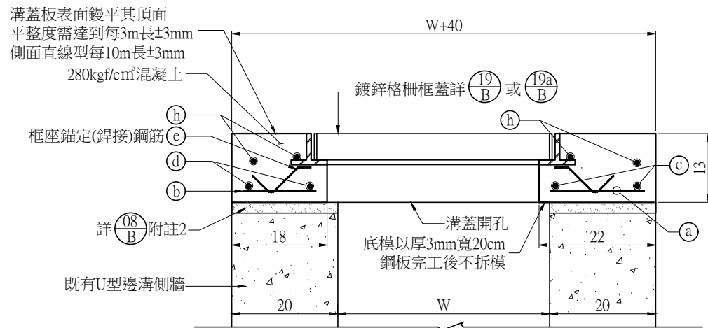
S 2型場鑄溝蓋板詳圖(板厚13cm) A1 (1:5) A3 (1:10) Unit:cm
