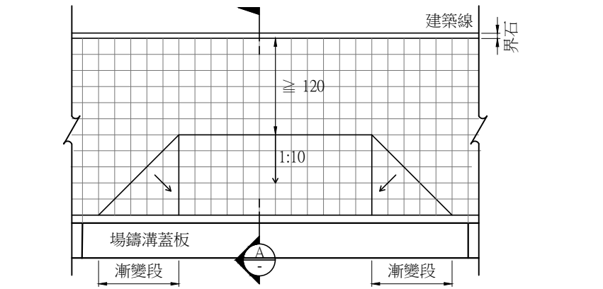
適用條件：人行道高度10cm時，人行道(包含設施帶)寬度 \geq 2.2\text{m} ， 人行道高度15cm時，人行道(包含設施帶)寬度 \geq 2.7\text{m} 。 橫越人行道之車行斜坡道平面圖(人行道寬度足夠時) NTS Unit:cm
