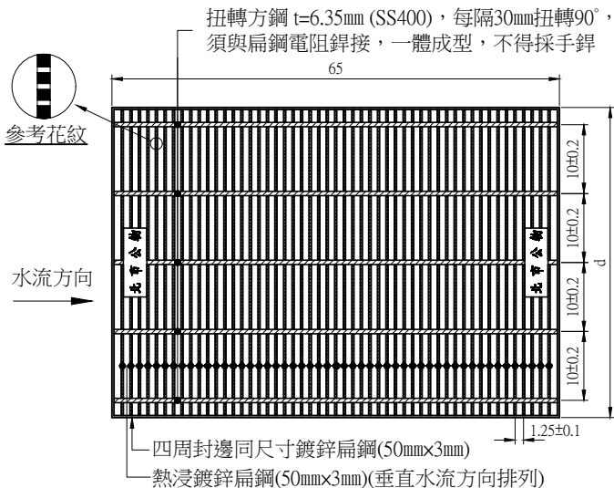
熱浸鍍鋅格柵蓋詳圖(人行道) Unit:cm
