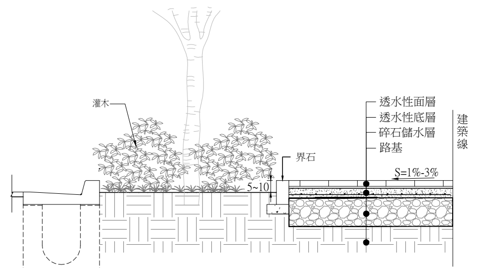
人行道透水鋪面(有植栽帶)斷面圖 NTS Unit:cm
