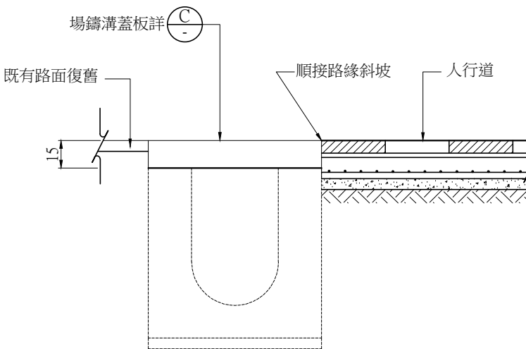
S 1型場鑄溝蓋板銜接人行道示意圖 Unit:cm
