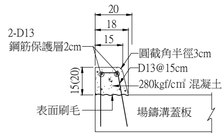
場鑄緣石配筋圖 A1 (1:10) A3 (1:20) Unit:cm
