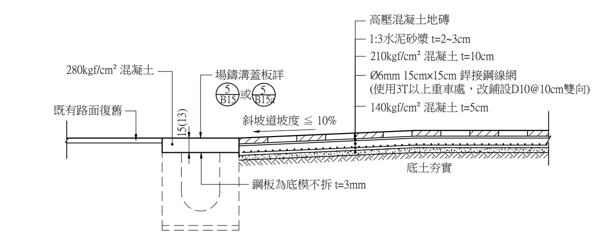
剖面圖 A1 (1:20) A3 (1:40) Unit:cm
