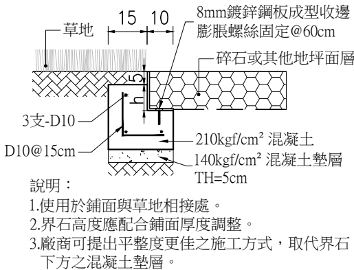
鋪面收邊詳圖(二) NTS Unit:cm ③
