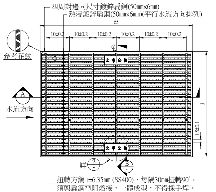
熱浸鍍鋅格柵蓋詳圖(路緣斜坡道) Unit:cm
