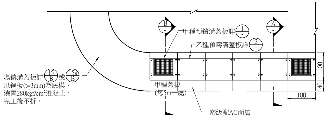
箱涵式側溝(預鑄溝蓋版)平面圖 A1 (1:40) A3 (1:80) Unit:cm
