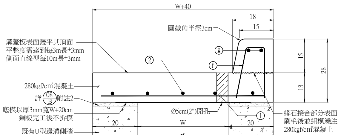
L 1型場鑄溝蓋板剖面圖(板厚13cm) A1 (1:5) A3 (1:10) Unit:cm
