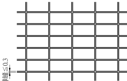
高壓混凝土磚鋪面平面圖(硬底層) A1 (1:10) A3 (1:20) Unit:cm
