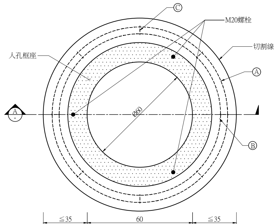
混凝土人孔框座平面圖 (Ø60cm人孔框蓋)
