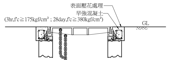
完成示意圖(四) 9 NTS
