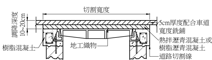
人手孔蓋降埋路面以下示意圖
