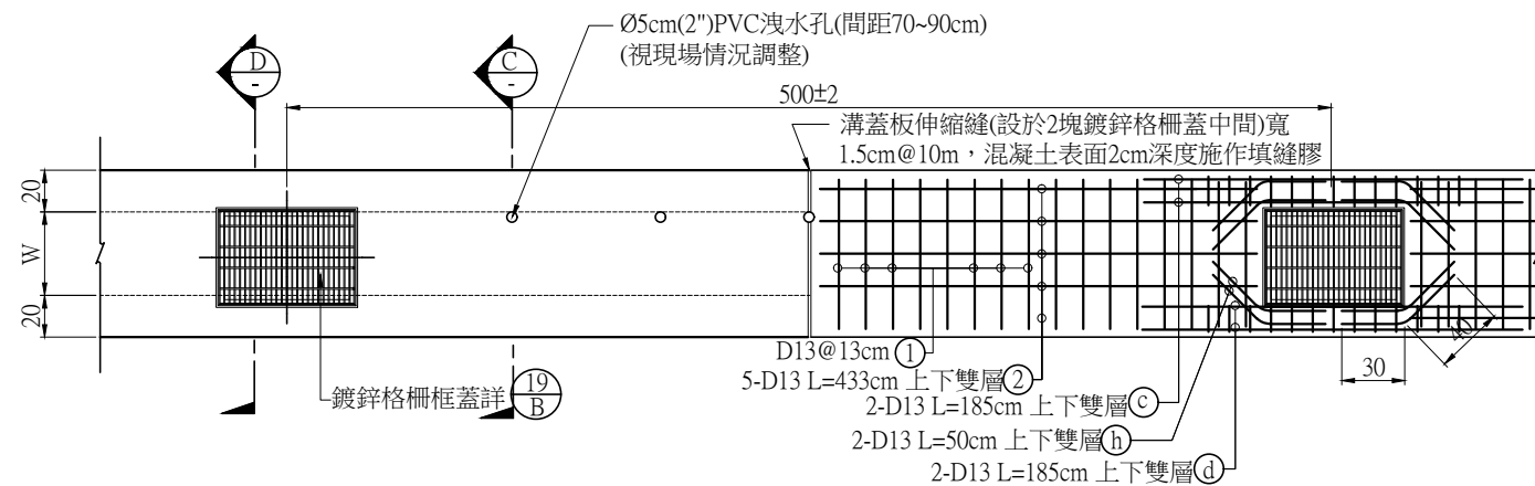
S型溝蓋板平面及鋼筋配置詳圖(板厚15cm) A1 (1:20) A3 (1:40) Unit:cm
