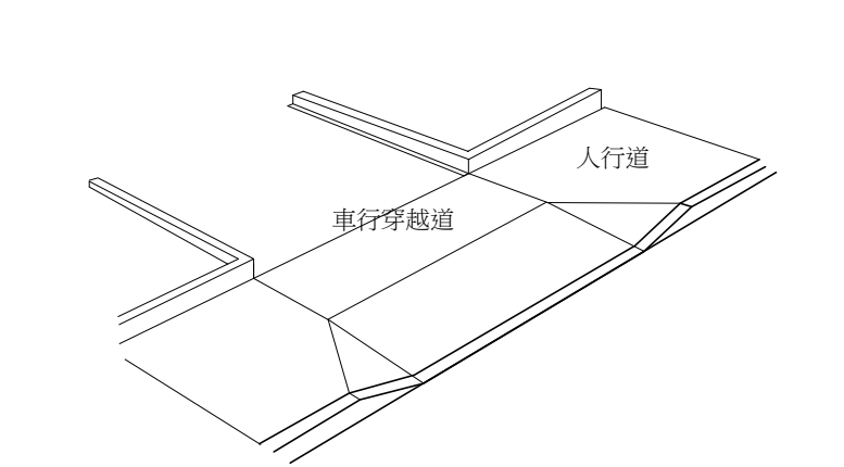
橫越人行道之車行斜坡道示意圖(人行道寬度足夠時) NTS
