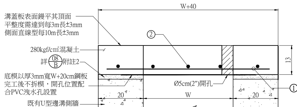
S 1型場鑄溝蓋板詳圖(板厚13cm) A1 (1:5) A3 (1:10) Unit:cm
