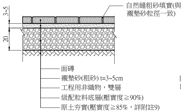
鋪面剖面圖(軟底層) A1 (1:10) A3 (1:20) Unit:cm
