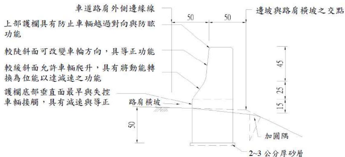
剖面圖
