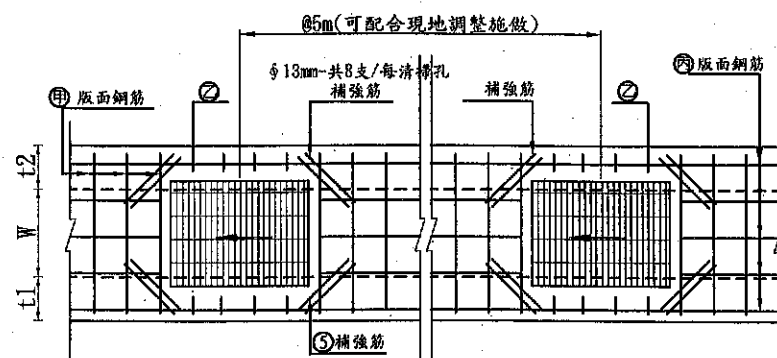
排水溝版面鋼筋(有清掃孔)示意圖
