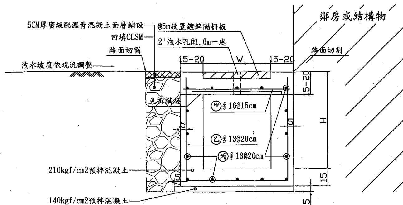
矩形溝標準圖 S=1/20
