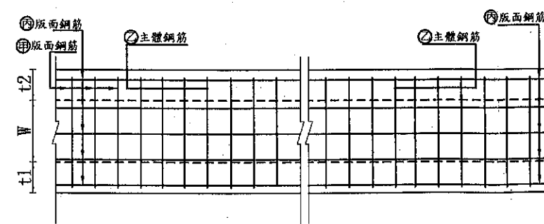
排水溝版面鋼筋(無清掃孔)示意圖
