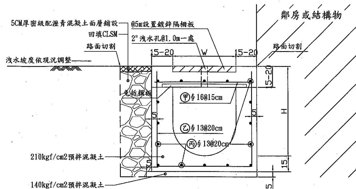
U形溝標準圖 S=1/20
